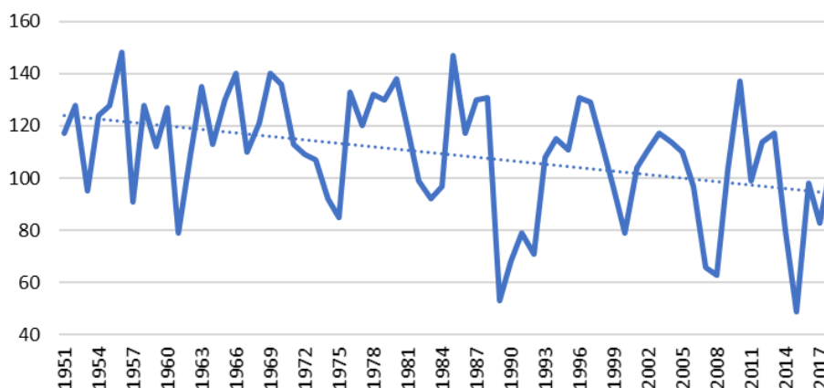
Päevi alla 0°C, Ristna
